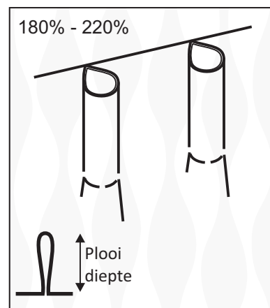
Vliesband, Kokerplooi
